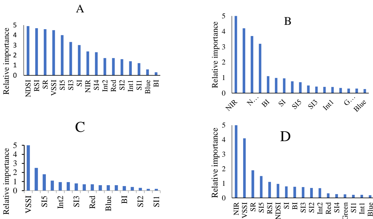
شکل ۲- اهمیت نسبی باندهای اصلی و شاخص‌های شوری در تخمین قابلیت هدایت الکتریکی عصاره اشباع خاک با استفاده از: الف) مدل درخت تصمیم و تصاویر لندست ۸ در فصل زمستان؛ ب) مدل جنگل تصادفی و تصاویر لندست ۸ در فصل تابستان؛ ج) مدل شبکه عصبی مصنوعی و تصاویر سنتینل ۲ در فصل زمستان؛ د) مدل جنگل تصادفی و تصاویر سنتینل ۲ در فصل تابستان
