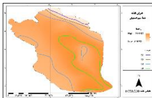
شکل ۷- دمای شهر اصفهان (منبع: نگارندگان، ۱۴۰۲)
