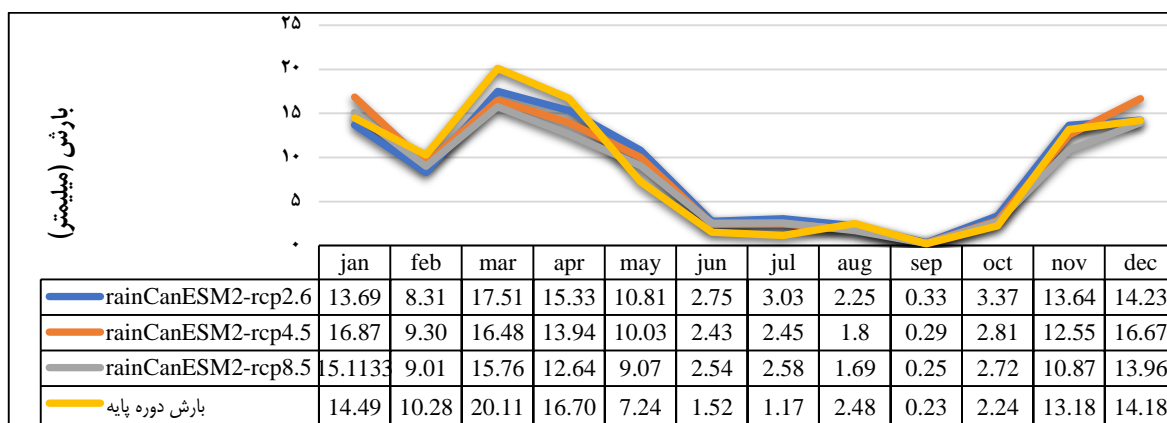
نمودار ۴- مقایسه بارش در آینده دور با دوره پایه در ایستگاه اصفهان (۲۰۵۱-۲۰۸۰)
