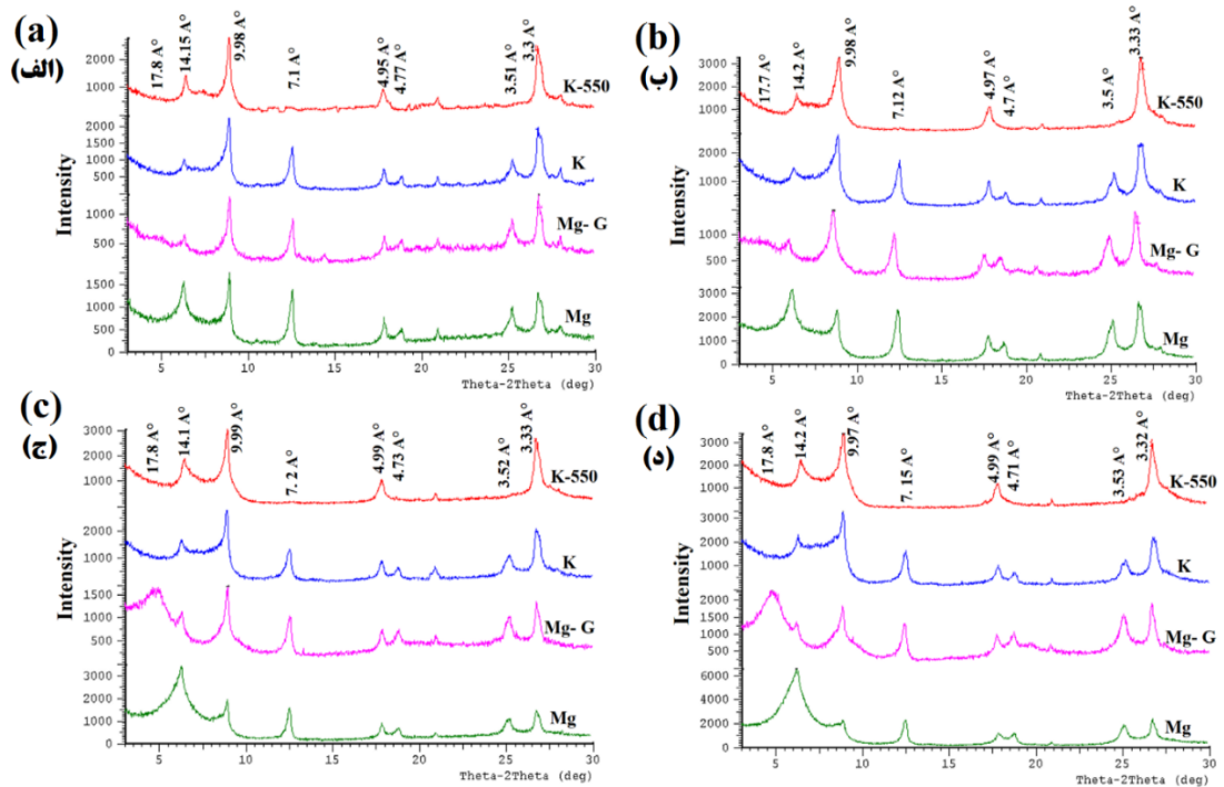
شکل ۲- دیفراکتوگرامهای اشعه X تعدادی از خاکهای مورد مطالعه. الف) افق Ap پروفیل ۱، ب) افق C1 پروفیل ۲، و ج) افق Btk4 پروفیل ۵، و د) افق Btk5 پروفیل ۶
