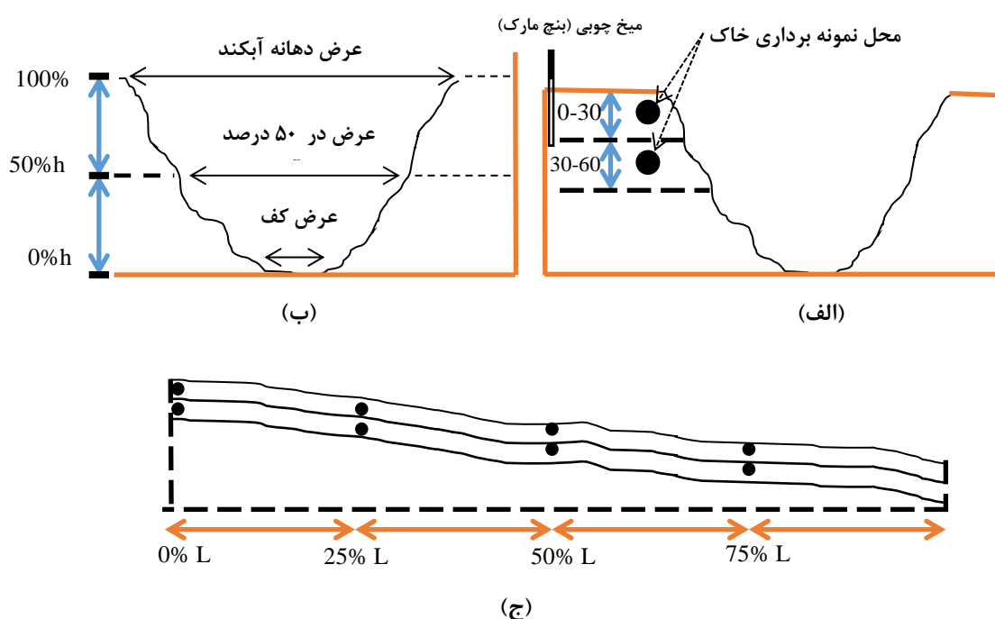
شکل ۲- الف) نمونه برداری خاک و ب) اندازه‌گیری عرض و عمق مقطع خندق و ج) نقاط اندازه‌گیری و نمونه‌برداری در طول خندق
