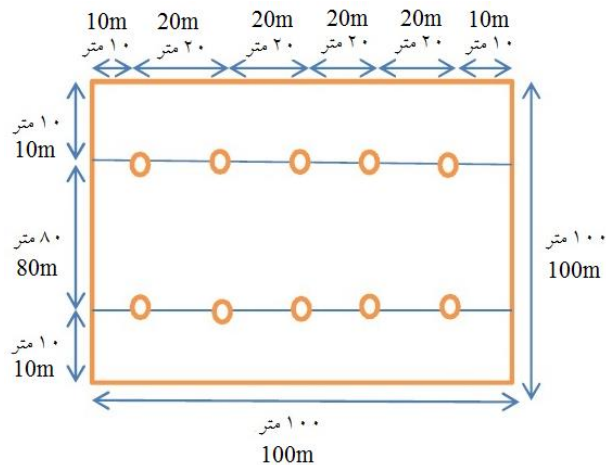
شکل ۱- طرح شماتیک محل و فواصل (بدون مقیاس) نمونه‌برداری خاک در توده‌های جنگلی مورد مطالعه
