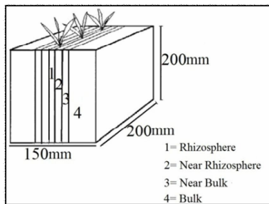
شکل (۱). طرح شماتیک سیستم جعبه ریزوسفر مورد استفاده
