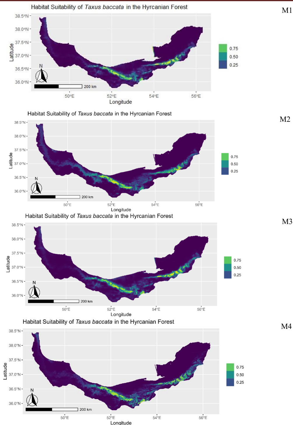
شکل ۲- نقشه پراکنش سرخدار با مدل MAXENT با متغیرهای مختلف (M1: ۱۹ متغیر زیست اقلیمی، M2: ۱۹ متغیر زیست اقلیمی و ۹ متغیر توپوگرافی، M3: ۱۹ متغیر زیست اقلیم و ۷ متغیر خاک، M4: ترکیب همه متغیرها با حذف همبستگی)
